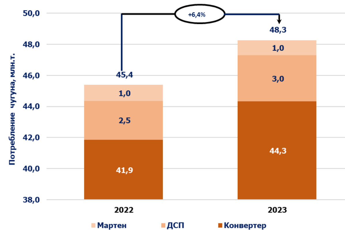
Динамика изменения потребления чугуна для выплавки стали
